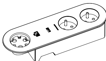
2 × 230V USB-A | LAN Cat6A | cable grommet
