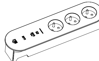
3 × 230V | USB C/A USB-A | LAN Cat6A
