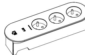
3 × 230V USB-A | LAN Cat6A
