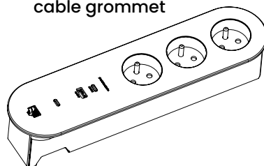
3 × 230V | USB C/A USB-C | LAN Cat6A
