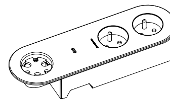
2 × 230V USB-C | cable grommet
